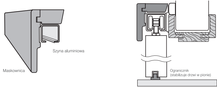
Przekrój pionowy systemu przesuwnego
