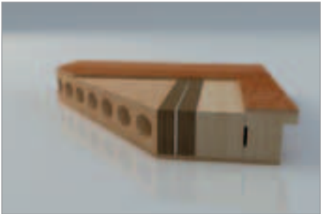
Wzmocniona konstrukcja drzwi o gr. 46 mm + płaskowniki stalowe
